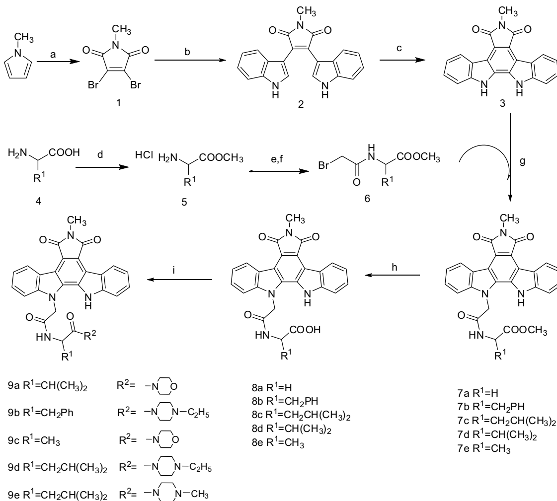
Scheme 1. The Synthesis of indolocarbazole analogs. Reagents and conditions: (a) \text{Br}_2 , -78^\circ\text{C} , \text{HNO}_3 ; (b) \text{CH}_3\text{CH}_2\text{Br} , \text{Mg} , \text{THF} , \text{indole} , \text{toluene} ; (c) \text{DDQ} , \text{toluene} ; (d) \text{Dry HCl} , \text{CH}_3\text{OH} ; (e) 10\%\text{NaOH} , \text{CH}_2\text{Cl}_2 ; (f) \text{BrCH}_2\text{COBr} , \text{TEA} ; (g) \text{NaH} , \text{DMF} ; (h) \text{NaH} , \text{DMF} ; (i) \text{CDI} , \text{R}_2\text{H} , \text{THF} .
